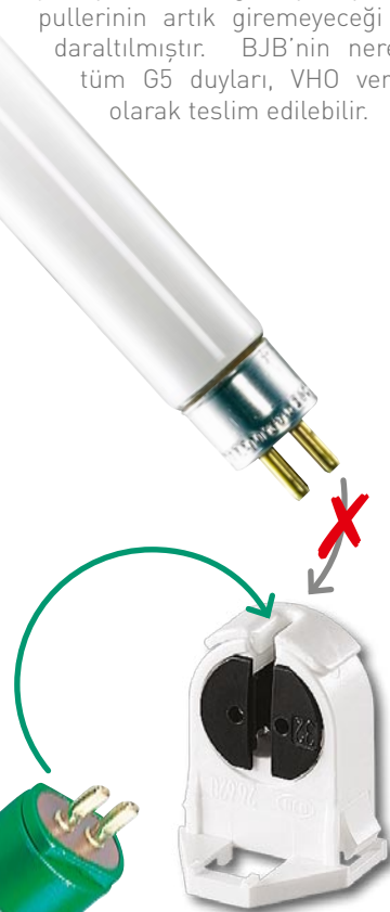
Philips MASTER TL5 VHO ampulleri için GX5 duy sistemi Yerleştirme aralığı, yuvarlak pinli T5 ampullerin takılmayacağı kadar daraltılmaktadır
